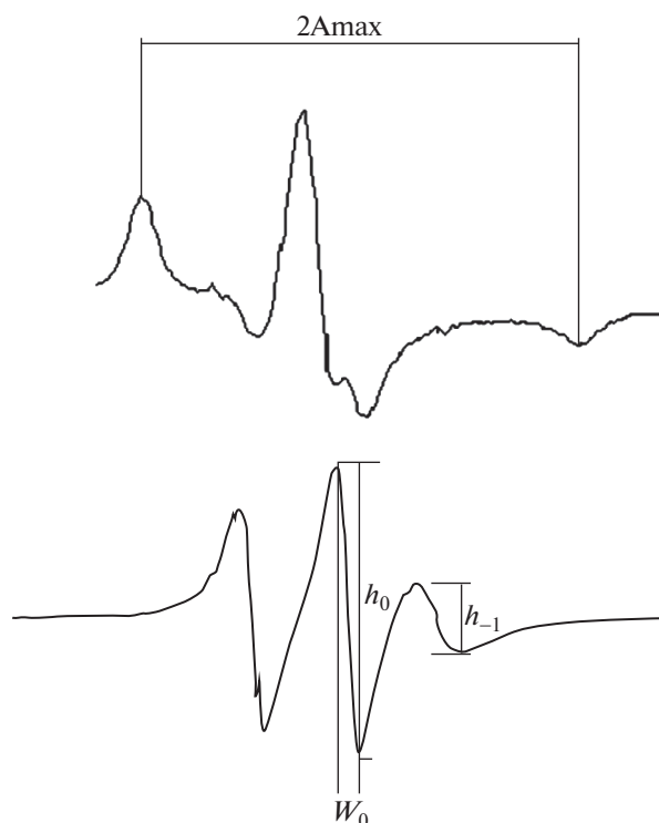
Рис. 12. Типичный ЭПР-спектр 5-ДСК и 16-ДСК меченных липосом из дипальмитоилфосфатидилохолина.
