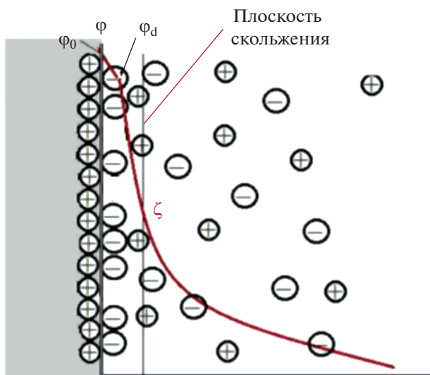
Рис. 3. Строение двойного электрического слоя: потенциал в плоскости скольжения соответствует электрокинетическому ζ-потенциалу везикулы. На рисунке ϕ 0 – потенциал стенки, ϕ d – Штерновский потенциал.
