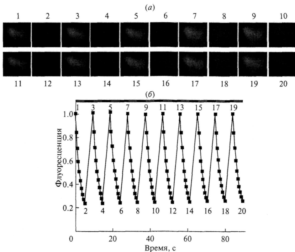
Рис. 3. Фотоконверсия KFP-НС в живых клетках млекопитающих. (а) Микрофотографии двух клеток линии Phoenix Eco, содержащих KFP-НС, полученные с использованием наборов фильтров TX2 для визуализации флуоресценции в красной области спектра. Фотографии получены последовательно в указанном порядке, каждое нечетное изображение соответствует KFP-НС в активированном состоянии, каждое четное – в потушенном состоянии. Тушение KFP-НС осуществлялось облучением зеленым светом (набор фильтров TX2), активация – облучением синим светом (набор фильтров GFP). (б) Изменение интенсивности флуоресценции KFP-НС в клетках, показанных на панели а. Серые и черные прямоугольники над графиком обозначают интервалы облучения зеленым и синим светом, соответственно. Цифры соответствуют изображениям на панели а.
